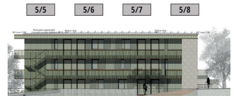
Haus 5 Ansicht Nord
